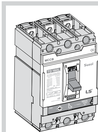
Автоматический выключатель Circuit breaker
