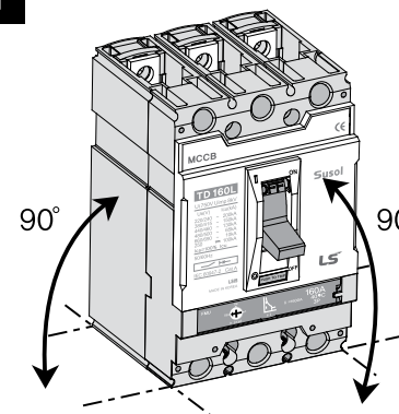
Автоматический выключатель Circuit breaker
